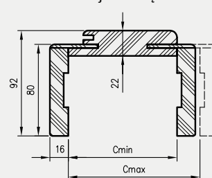
Przekrój OR z kątem T80
