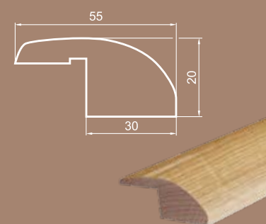
Listwa progowa
